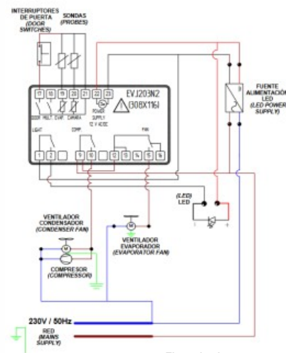
Ejemplo de esquema eléctrico.
