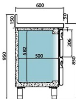
BM 1/2 x 200
