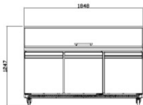
ALZADO/ ELEVATION/ VUE LATÉRAL
