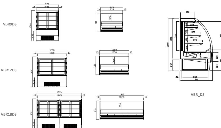
ALZADO
