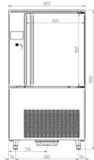
ALZADO/ ELEVATION/ VUE LATÉRAL
