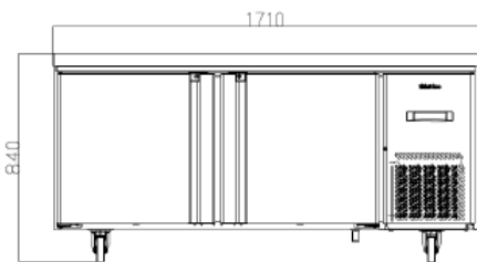
MR67BT
