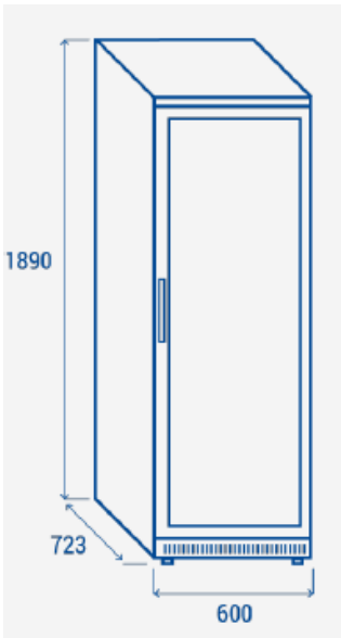
RV400GD
