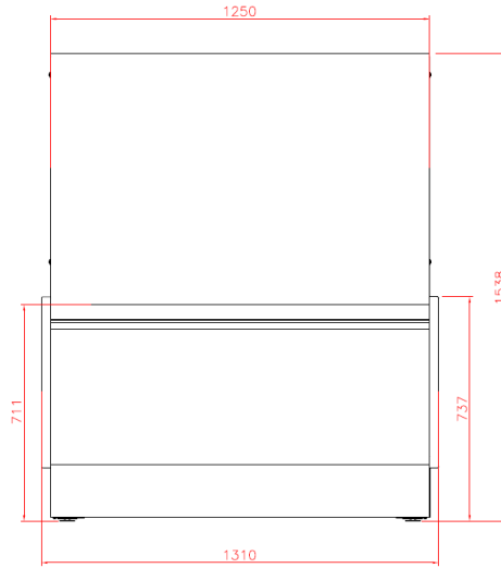
VLY12 V
