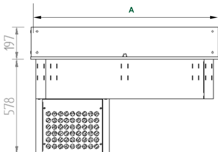
Alzado / Elevation / Vue Latéral
