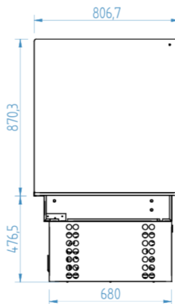
Perfil / Right View / Vue de Profil
