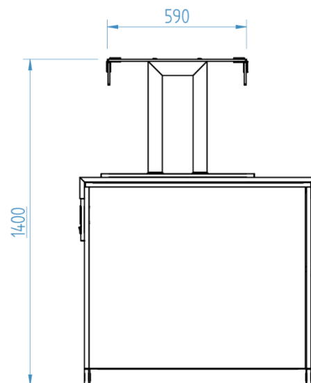
Perfil / Right View / Vue de Profil
