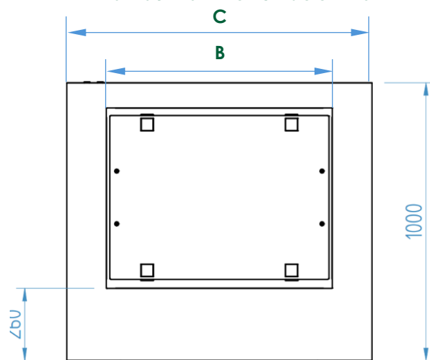
Planta / Plan View / Vue en Plan
