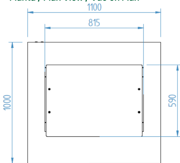
Planta / Plan View / Vue en Plan
