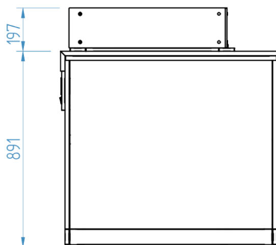
Perfil / Right View / Vue de Profil
