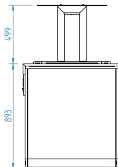
Perfil / Right View / Vue de Profil
