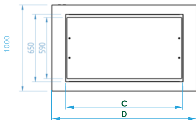
Planta / Plan View / Vue en Plan
