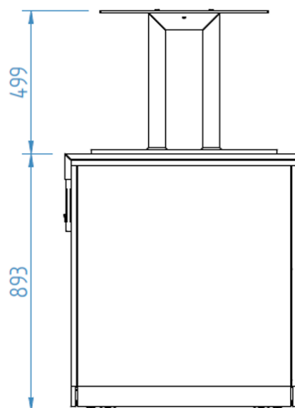
Perfil / Right View / Vue de Profil
