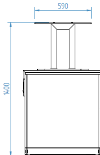
Perfil / Right View / Vue de Profil
