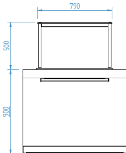
Alzado / Elevation / Vue Latéral
