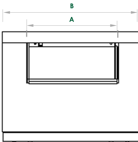
Alzado / Elevation / Vue Latéral
