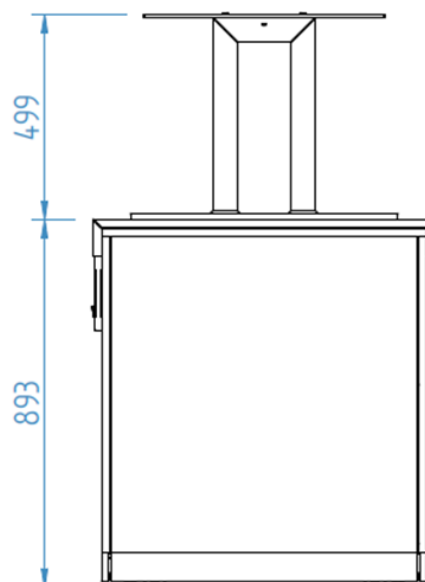
Perfil / Right View / Vue de Profil
