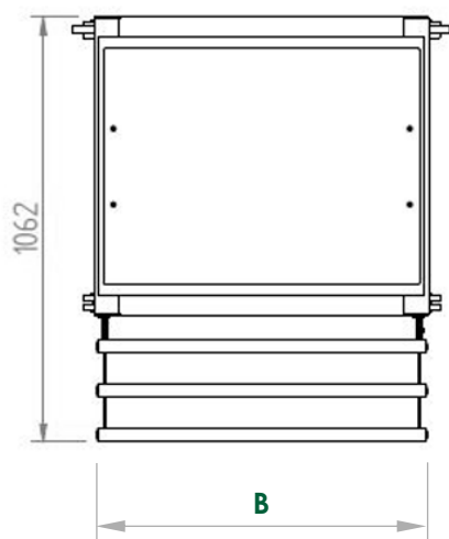
Planta / Plan View / Vue en Plan
