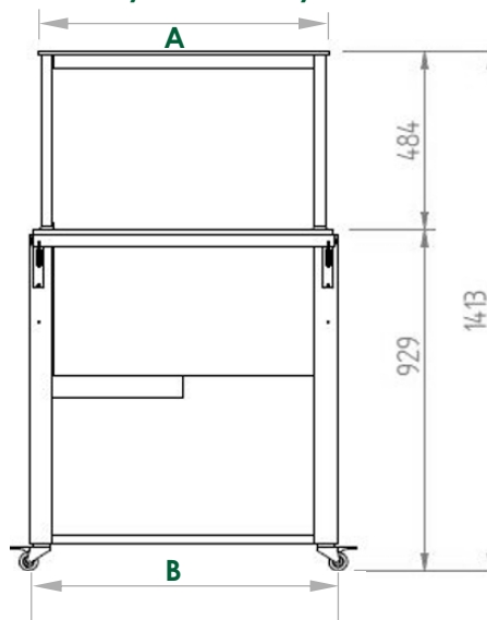
Alzado / Elevation / Vue Latéral
