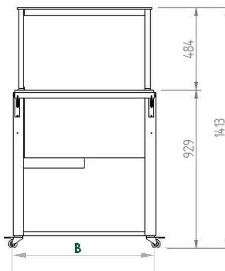
Alzado / Elevation / Vue Latéral
