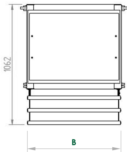
Planta / Plan View / Vue en Plan
