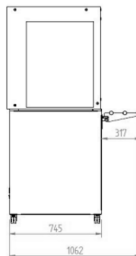
Perfil / Right View / Vue de Profil
