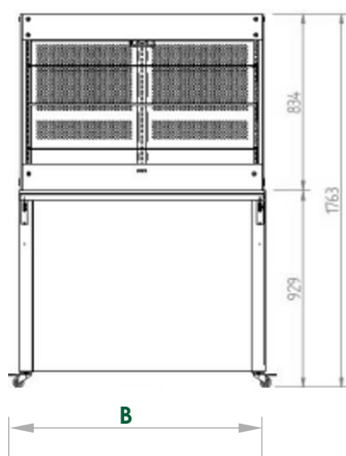
Alzado / Elevation / Vue Latéral
